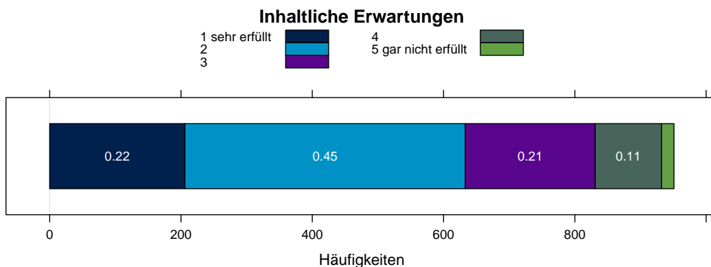
Abbildung 4: Inhaltliche Erwartungen
